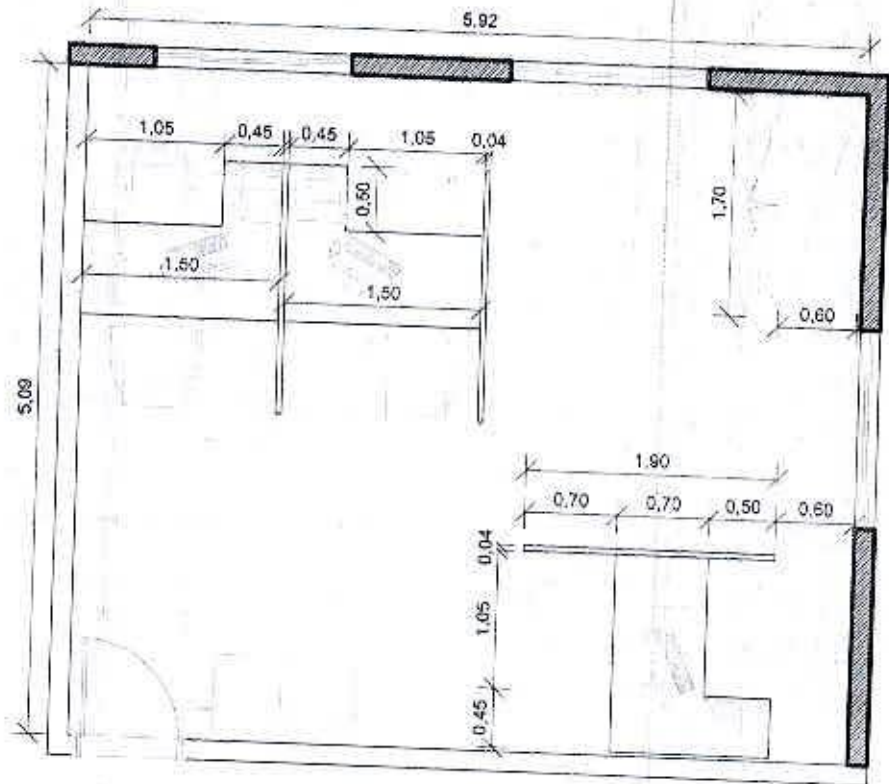
1 Planta Baixa 1 : 50
