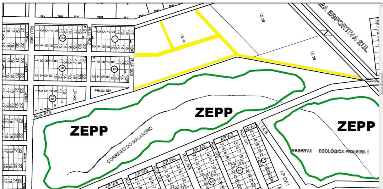
03) ALINHAMENTO DE RUAS URBANAS COM APLICAÇÃO DE ESTACAS NUMERADAS, DE 10 EM 10 MT NAS LATERAIS E BALIZAS DE 20 EM 20 MT NO EIXO DA RUA, BALIZANDO DE ACORDO COM CROQUI APRESENTADO. ( COLOCAR LARGURAS) E MAPAS EM AUTOCAD.
