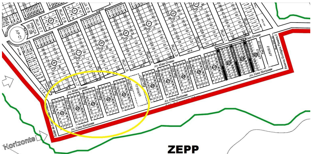
01) ALOCAÇÃO DOS LOTES EM ESCALAS, APLICAÇÃO DE MARCOS NUMERADOS E C/ PLOTAGEM TOPOGRAFICAS C/ COORDENADAS GEOGRAFICAS, MEMORIAL DESCRITIVO E MAPAS EM AUTOCAD.
