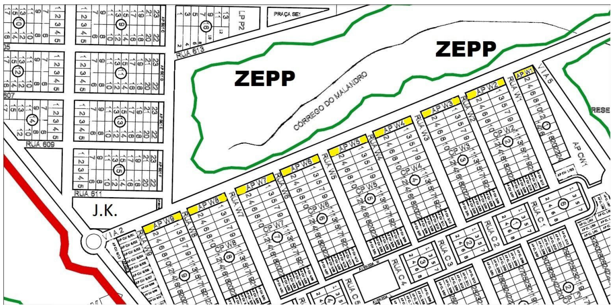
01) ALOCAÇÃO DOS LOTES EM ESCALAS, APLICAÇÃO DE MARCOS NUMERADOS E C/ PLOTAGEM TOPOGRAFICAS C/ COORDENADAS GEOGRAFICAS E MAPAS EM AUTOCAD.
